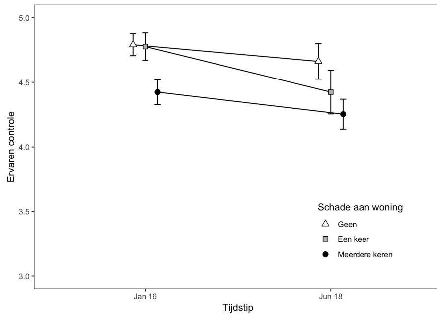
Figuur 5.5. Verandering van machteloosheid (boven) en ervaren controle (onder), als functie van het al dan niet hebben van schade, met 95% betrouwbaarheidsinterval.
